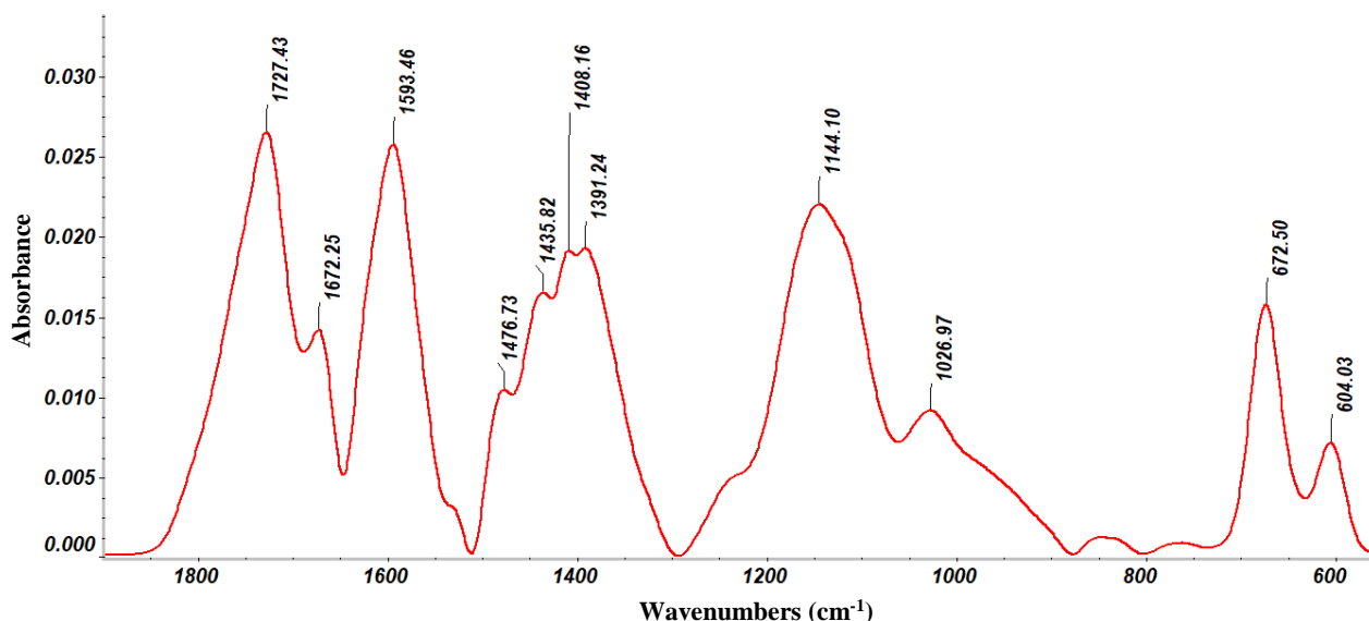
شکل ۹: طیف FTIR از محصولات خوردگی سبز رنگ طلایی کتیبه شومینه؛ ارتعاشات COO - در ۱۵۹۳cm -1 و ۱۴۰۸cm -1 قابل مشاهده است.
