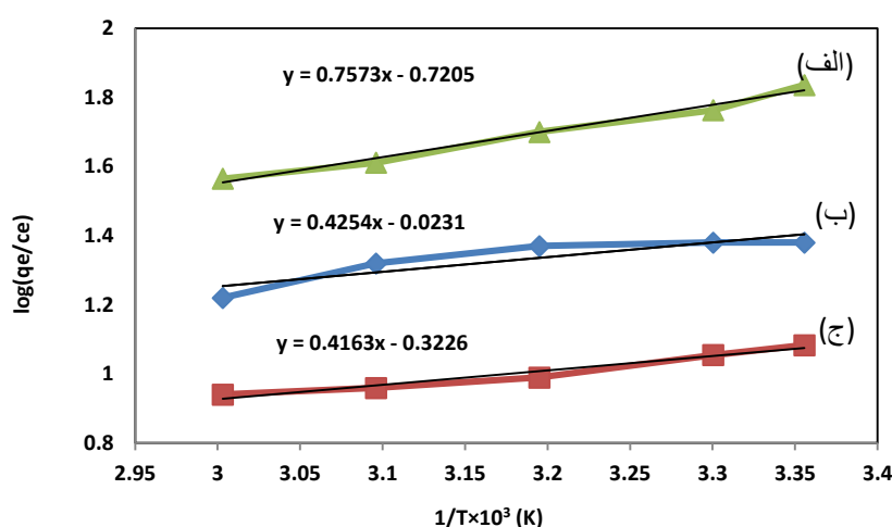
شکل ۱۹: نمودار ترمودینامیکی \log(q_e/c_e) برحسب 1/T(K) ، (الف) آلكالی آبی، (ب) اریوكرم سیاه T، (ج) هیدروکسی نفتول آبی.
