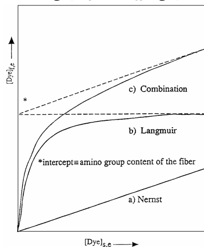
شکل ۱: ساز و کارهای متفاوت جذب پیشنهاد شده برای رنگزای الیاف نایلون با مواد رنگزای آنیونیکی [۴]. (محور عمودی غلظت رنگزا در فاز لیف و محور افقی غلظت رنگزا در فاز محلول را نشان می‌دهد).
