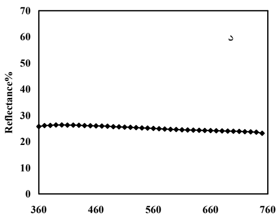
شکل ۴: طیف انعکاسی نمونه‌های سنتز شده: الف) نمونه آبی، ب) نمونه زرد، ج) نمونه ارغوانی و د) نمونه خاکستری.
