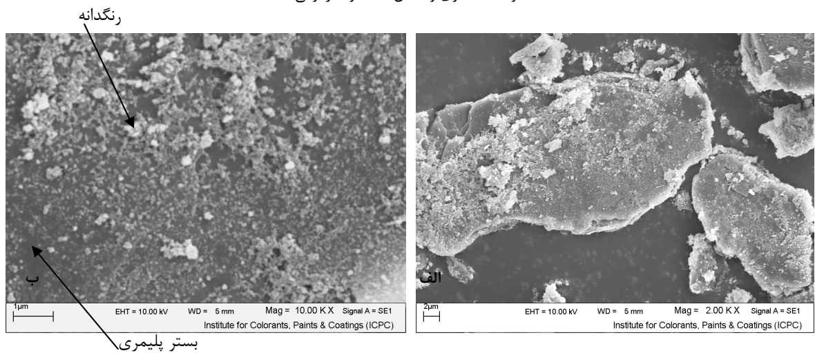
شکل ۲: تصویر میکروسکوپ الکترونی از سطح میکای پوشش داده شده، الف: نمای کلی پولک میکا و ب: نمای جزئی سطح میکا.
