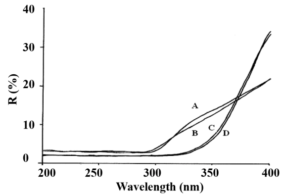
شکل ۳: طیف انعکاسی نمونه های پشمی در محدوده ۲۰۰ تا ۴۰۰ نانومتر (A نمونه خام (B نمونه اکسید شده (C نمونه عمل شده با 0.038 گرم بر لیتر دی اکسید تیتانیوم و (D BTCA نمونه عمل شده با 0.075 گرم بر لیتر دی اکسید تیتانیوم و BTCA).
