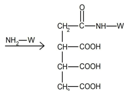
شکل ۴: مکانیزم اتصال BTCA به سطح پشم و ایجاد پیوندهای کووالانس (Cys: اسید آمینه سیستین، W: پشم).
