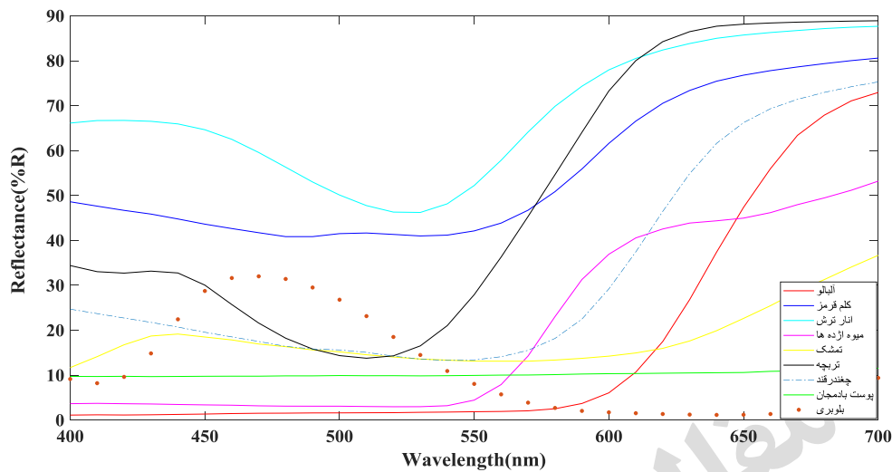
شکل ۱- منحنی انعکاسی ۹ فوتوآند حساس شده با مواد رنگزای طبیعی در محدوده طول موج مرئی.
