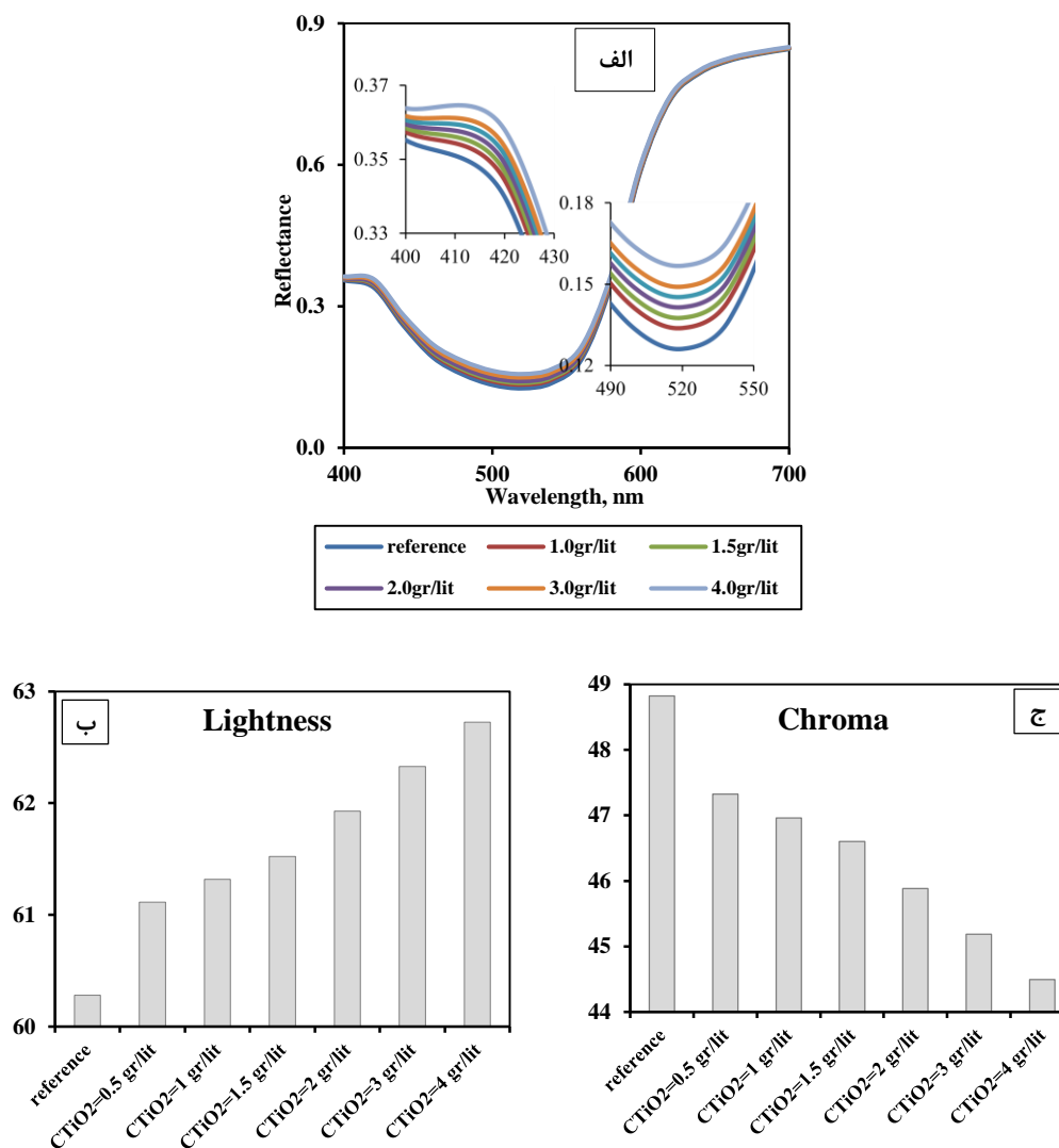
شکل ۵: (الف) طیف انعکاسی، (ب) روشنایی و (ج) خلوص نمونه‌های قرمز پوشش داده شده با ذرات دی اکسیدتیتانیوم به قطر ۱۲۰ نانومتر، شبیه‌سازی شده توسط مدل پیشنهادی.
