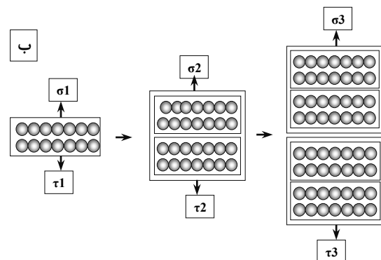
شکل ۱: الف) نمای شمایی از پدیده‌های انعکاس و انتقال از لایه سطحی الیاف و ب) نحوه شکل‌گیری لایه‌ها در مدل هندسی [۲۲].
