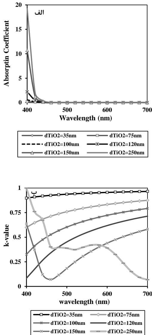
شکل ۴: (الف) ضریب جذب و (ب) ضریب k رنگدانه‌های دی‌اکسید تیتانیوم با قطر مختلف.
