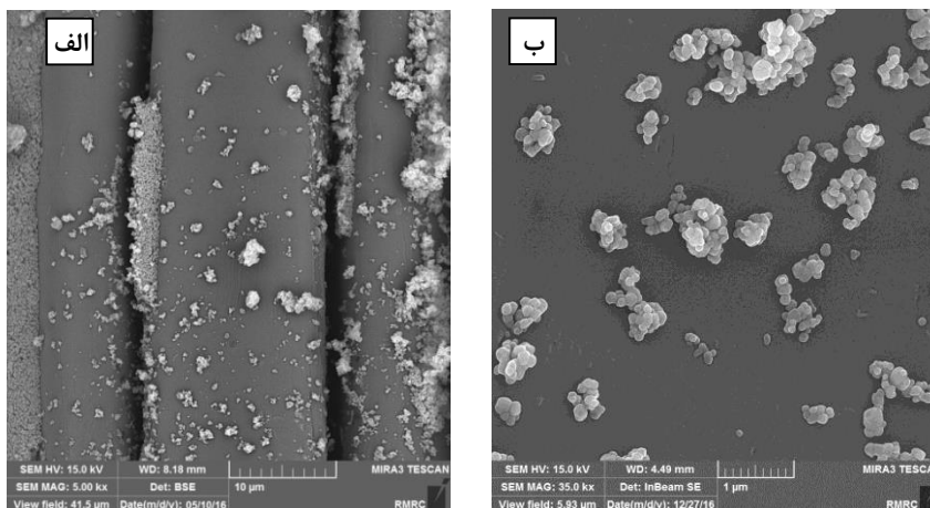
شکل ۶: تصاویر FESEM از پارچه پوشش داده شده با ذرات دی اکسیدتیتانیوم با قطر ۱۲۰ نانومتر و غلظت ۴ گرم برلیتر. (الف: بزرگ نمایی ۵۰۰۰ و ب: بزرگ نمایی ۱۵۰۰۰)
