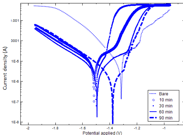
شکل ۳: منحنی‌های نمودار پلاریزاسیون نمونه‌های بدون پوشش و پوشش داده شده در محلول پوشش تبدیلی بر پایه وانادیم در pH=8، زمان‌های مختلف غوطه‌وری غلظت ۲۰ گرم بر لیتر از کلرید سدیم مورد استفاده و در دمای محیط.
