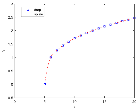
شکل ۱۵: برابری مشتق چپ و راست و تأثیر آن بر برازش اسپلاین استفاده شده به منظور محاسبه زاویه تماس. تصویر سمت راست) برازش منحنی اسپلاین بر سطح و قطره، تصویر سمت چپ) برازش منحنی اسپلاین بر پروفایل قطره.
