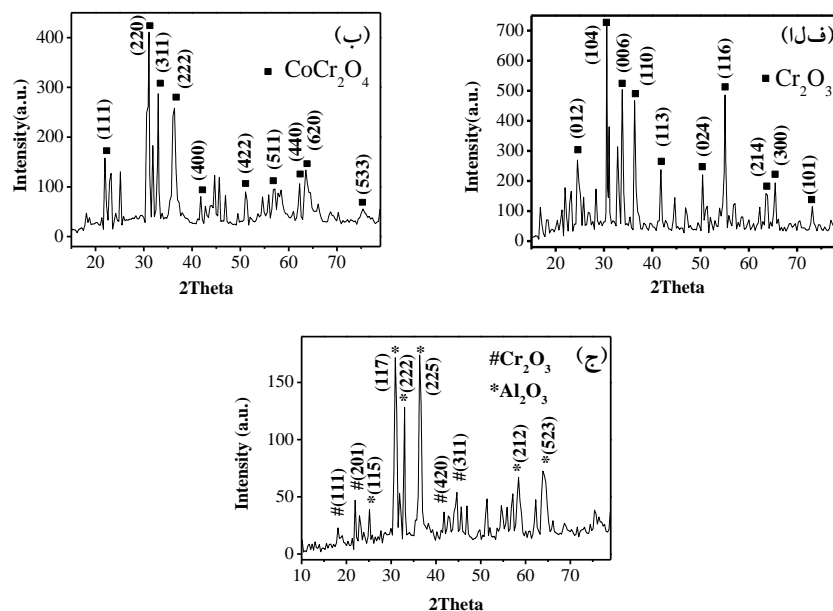
شکل ۴: طیف پراش پرتو ایکس نانورنگدانه‌های ساخته شده به روش هیدروترمال و پخت داده شده در 770^\circ C (الف) نمونه S1، (ب) S2 و (ج) S3.
