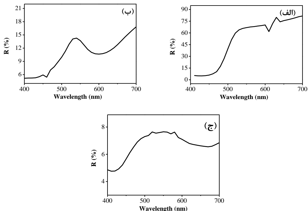
شکل ۷: طیف بازتاب نفوذی از سطح نانورنگدانه‌های ساخته شده به روش هیدروترمال و پخت داده شده در 770^{\circ}\text{C} (الف) نمونه S1، (ب) S2 و (ج) S3.
