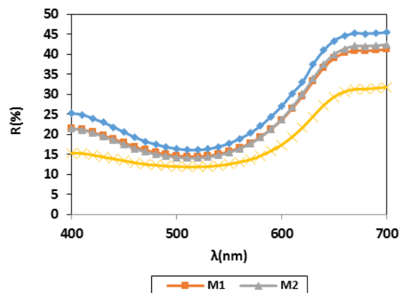
شکل ۷: طیف بازتاب نفوذی مربوط به رنگدانه‌ها.
