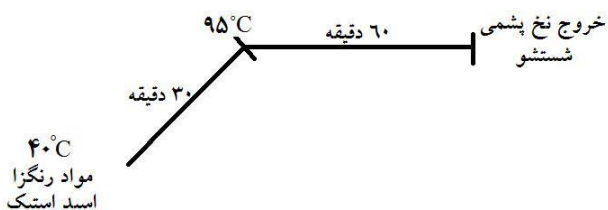
شکل ۳: گراف رنگری نخ پشمی.
