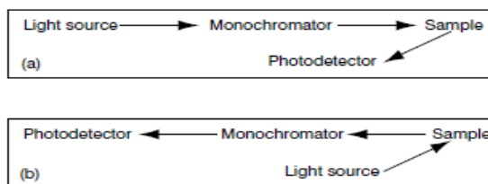
شکل ۶: شکل شمایی دو آرایش نوری متفاوت برای ابزارهای اندازه‌گیری رنگ [۶].
