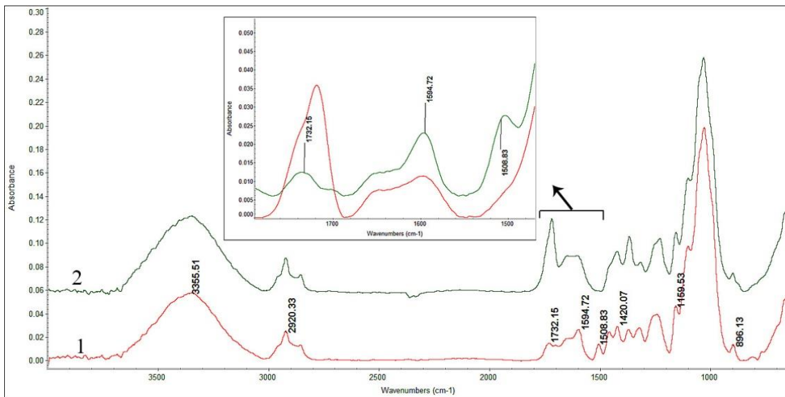
شکل ۵: مقایسه طیف ATR، (۱) چوب شاهد (Control) (۲) نمونه شاهد کهنگی تسریعی (W-UV).
