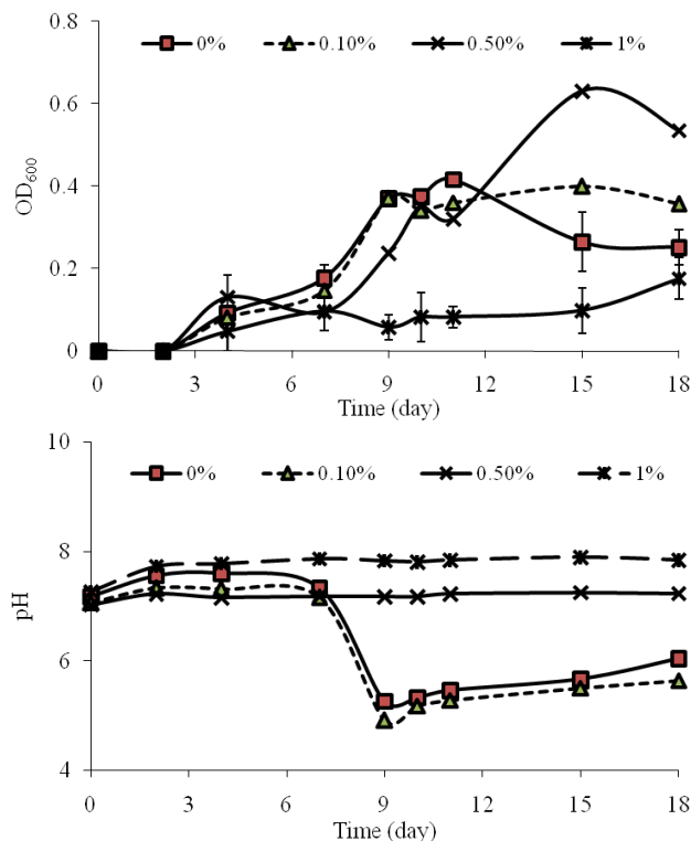
شکل ۴: تغییرات pH و کدورت محیط کشت با حضور باکتری تیوباسیلوس تیوپاروس و نمونه‌های سیمانی عاری و حاوی درصد‌های مختلف نانوذرات دی‌اکسید تیتانیم.
