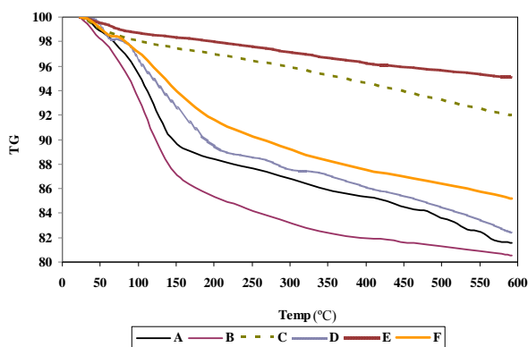
شکل ۶: تجزیه و تحلیل TG هیبریدهای مختلف (A زئولیت، B STZ0.2-0.4، C STZ0.2-0.4 (D، STZ0.2-0.2 (E، STZ0.4-0.2 (F و STZ0.4-0.4)
