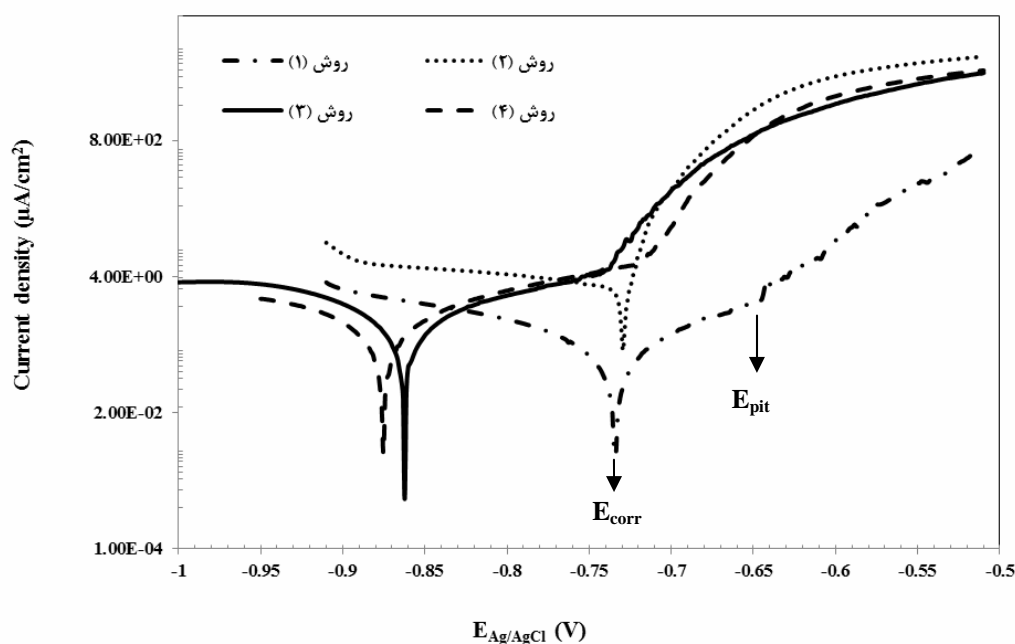
شکل ۱: نمودارهای پلاریزاسیون در محلول ۰.۵٪ وزنی NaCl پس از ۳۰ ثانیه غوطه‌وری در محلول نمکی برای نمونه‌های آماده‌سازی شده با روش‌های (۱): چربی‌گیری، (۲): شستشوی قلیایی، (۳): شستشوی قلیایی+شستشوی اسیدی و (۴): سنباده‌زنی+شستشوی قلیایی+شستشوی اسیدی.
