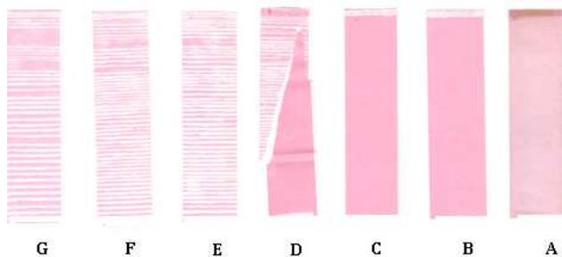
شکل ۸: مقایسه کنده شدن سطح کاغذهای شاهد و تیمار شده با روغن سنگین.
