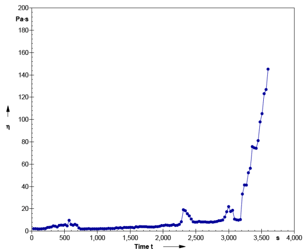
شکل ۱: تغییرات گرانروی پوشش ۱۰٪ نانورس و لاتکس.
