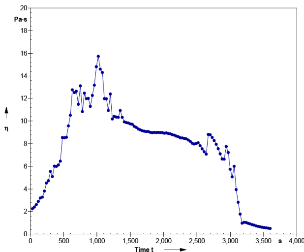
شکل ۲: تغییرات گرانروی پوشش ۵۰٪ کربنات کلسیم و لاتکس.
