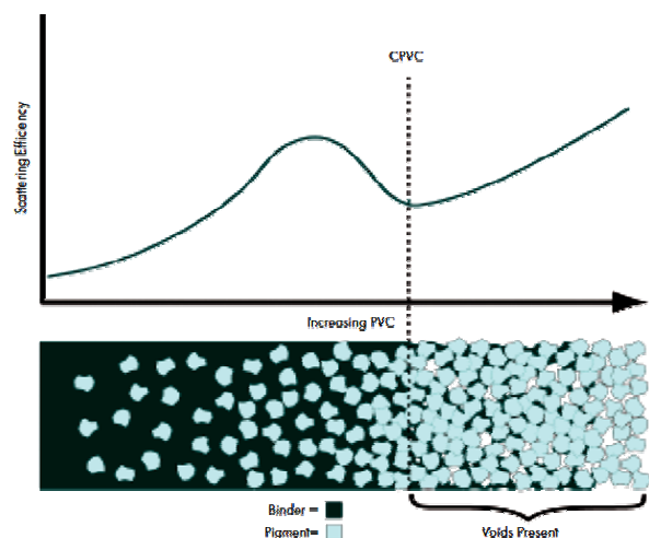
شکل ۴: وابستگی بازده پراکنش نور به غلظت حجمی رنگدانه [۲۸].
